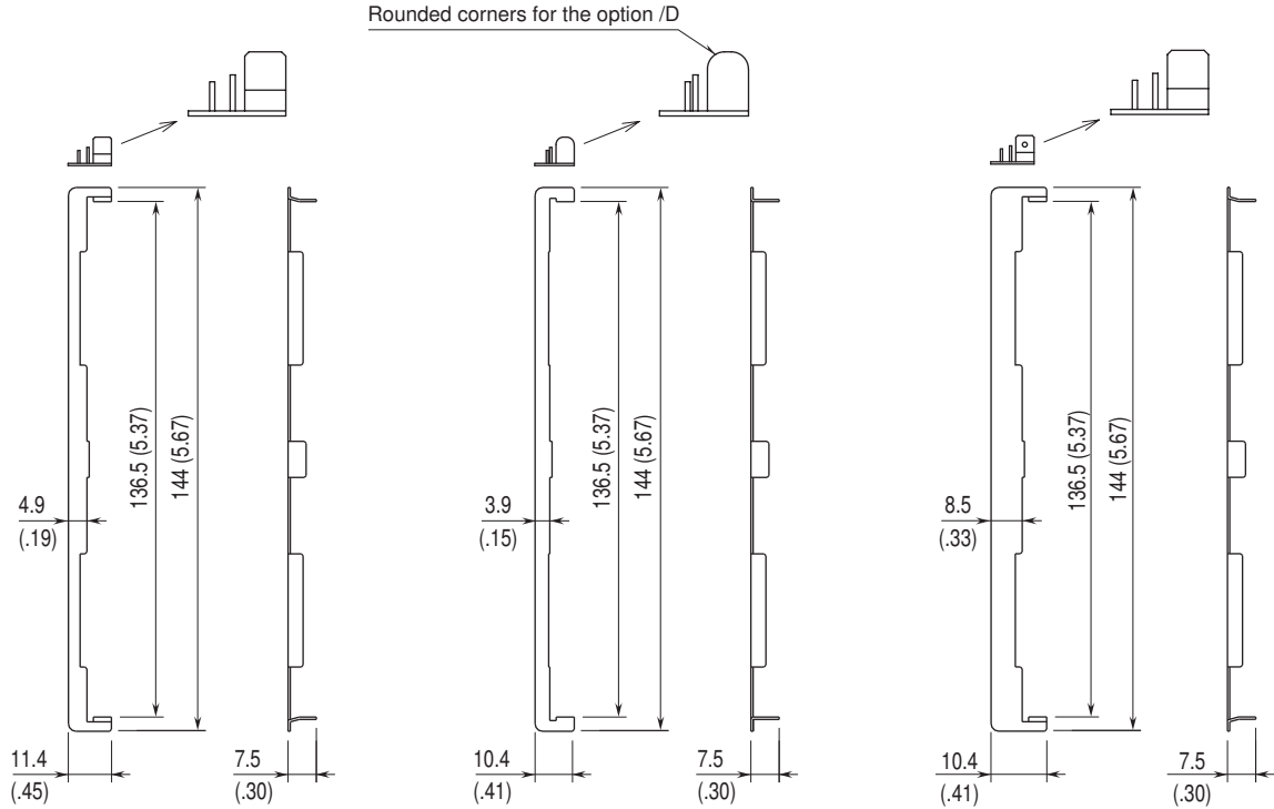
STANDARD BEZEL *2
