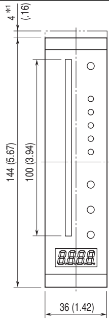
STANDARD BEZEL *2
